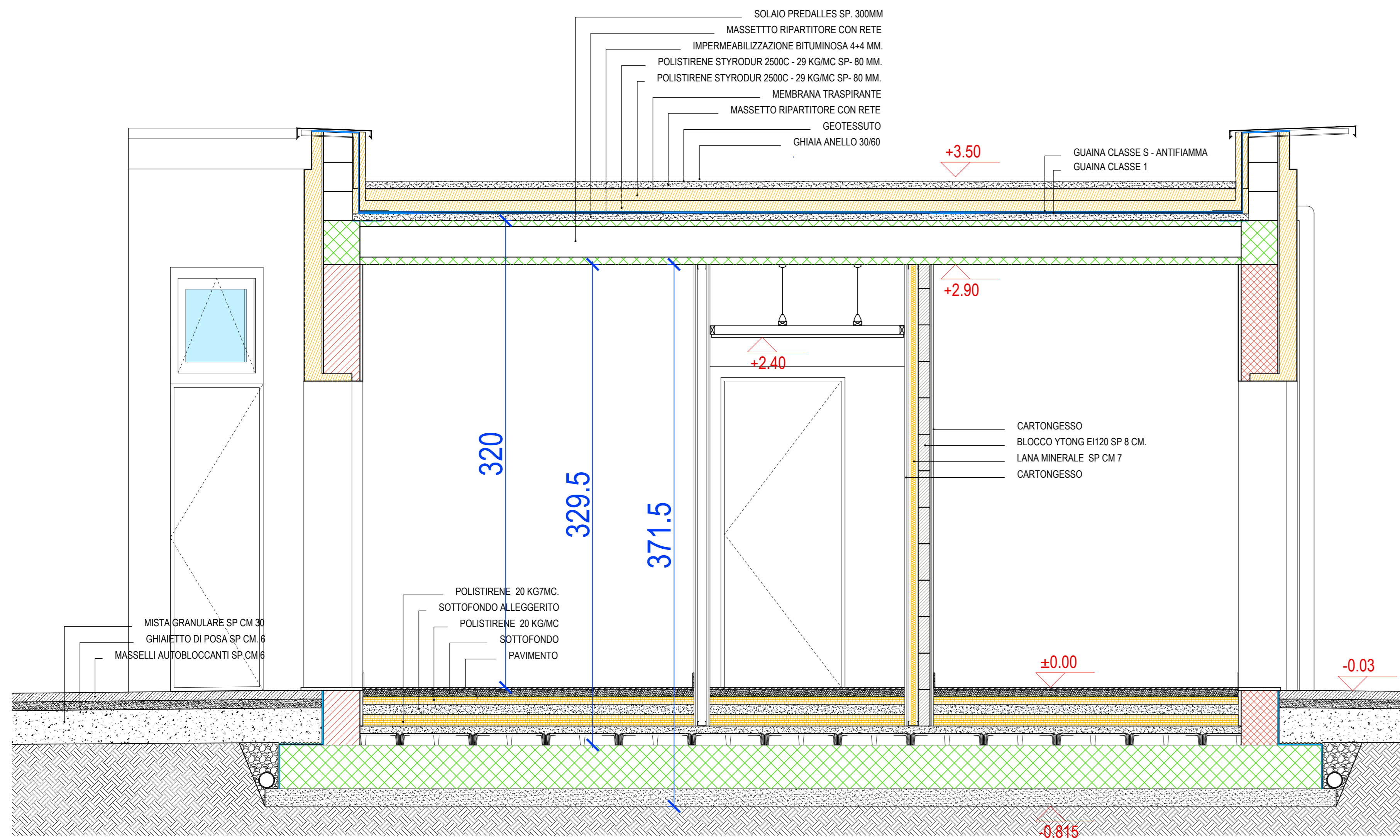
SEZIONE AA
