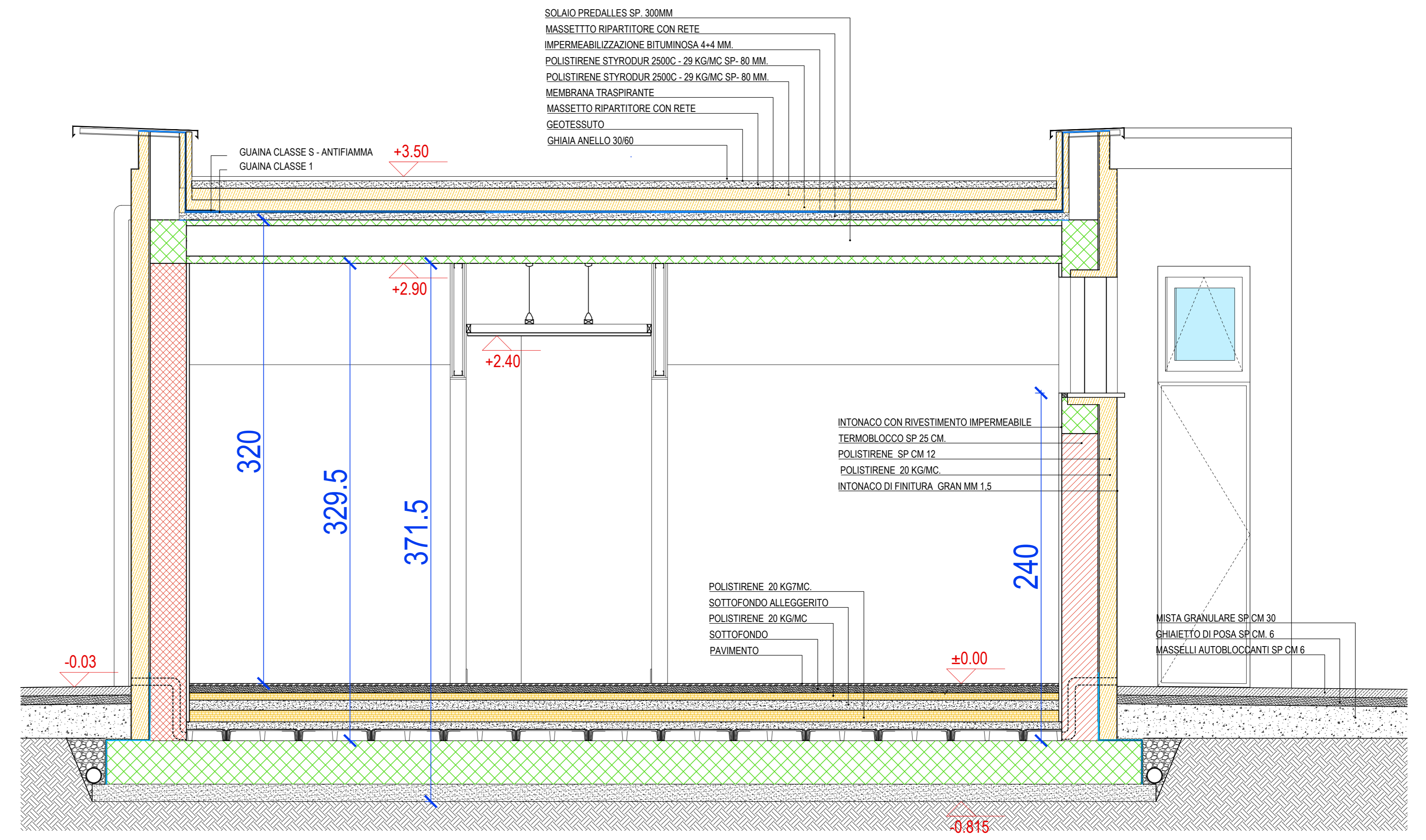
SEZIONE BB
