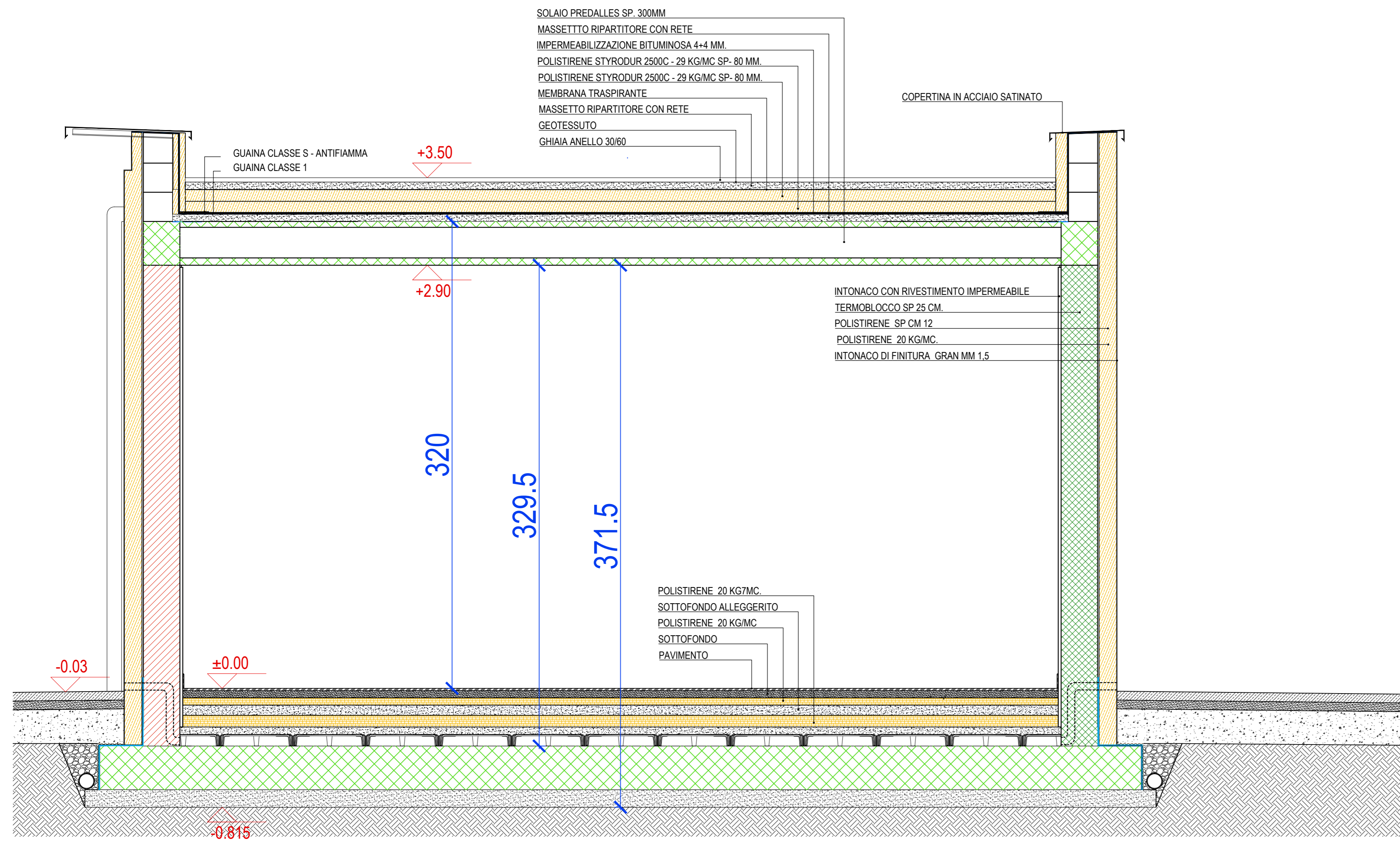
SEZIONE CC
